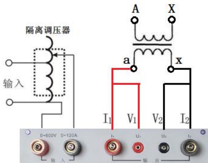
图 6-19 单相变压器空载试验接线图
