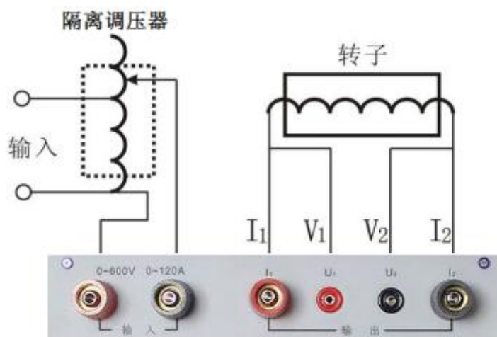
图 5-1 交流阻抗试验接线图
