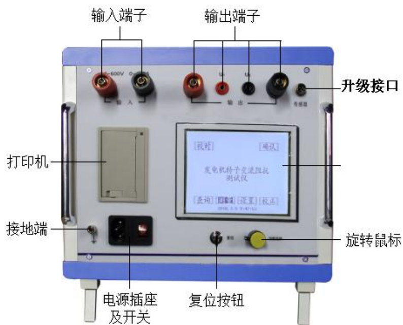
图 4-1 阻抗测试仪面板
