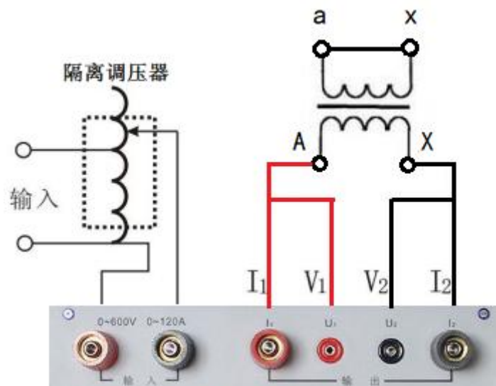
图 6-21 单相变压器短路试验接线图
